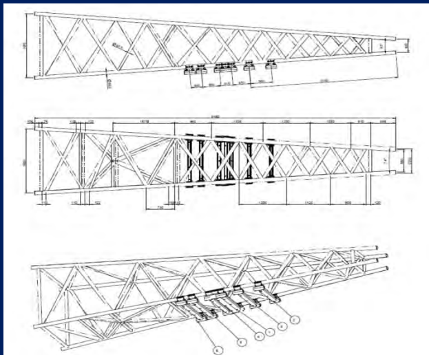
Fig 2. 6/10K Crane)
